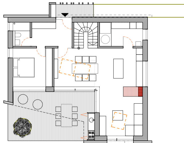
PRITLIČJE - tip 2 YEZIRA
